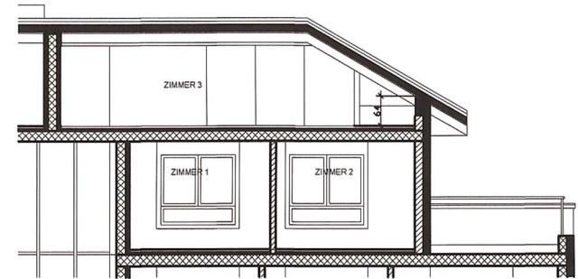
Schnitt A-A
